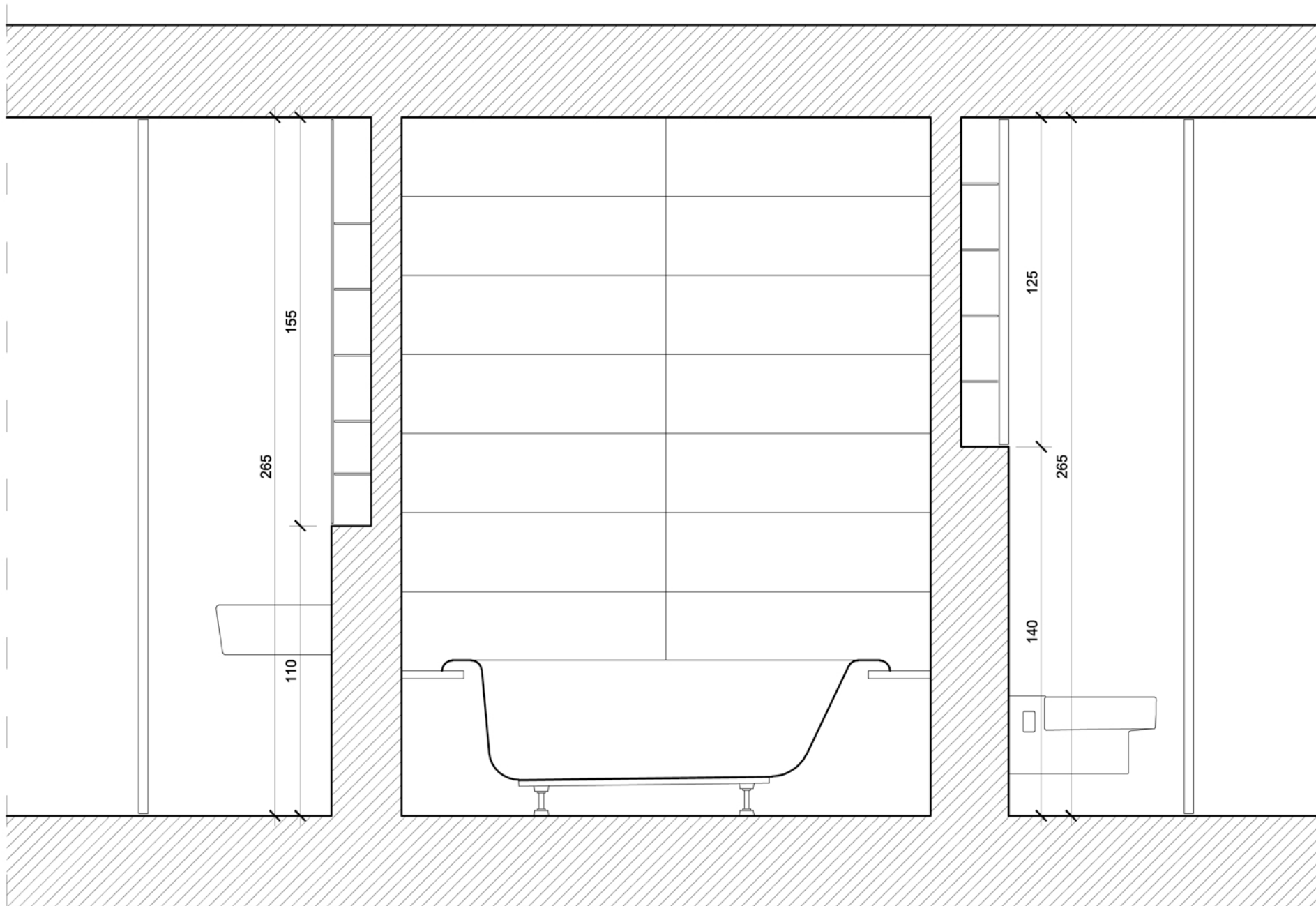
PRZEKRÓJ A-A
