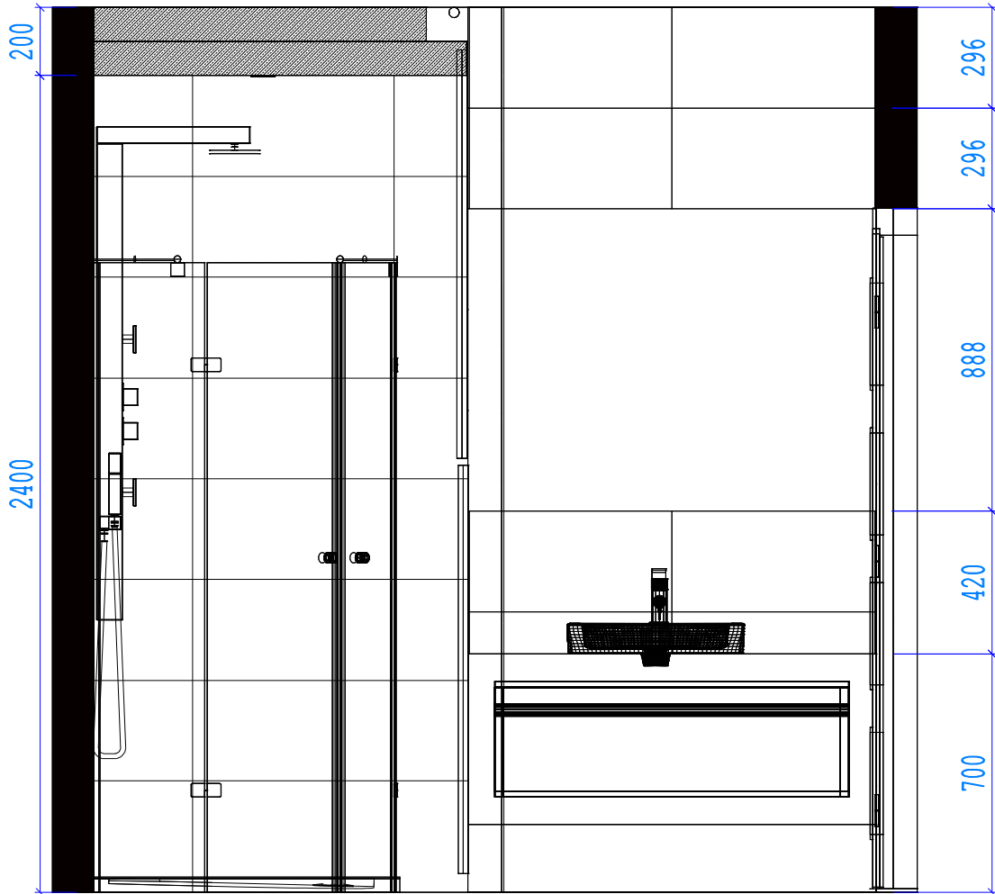
PRZEKRÓJ A-A
