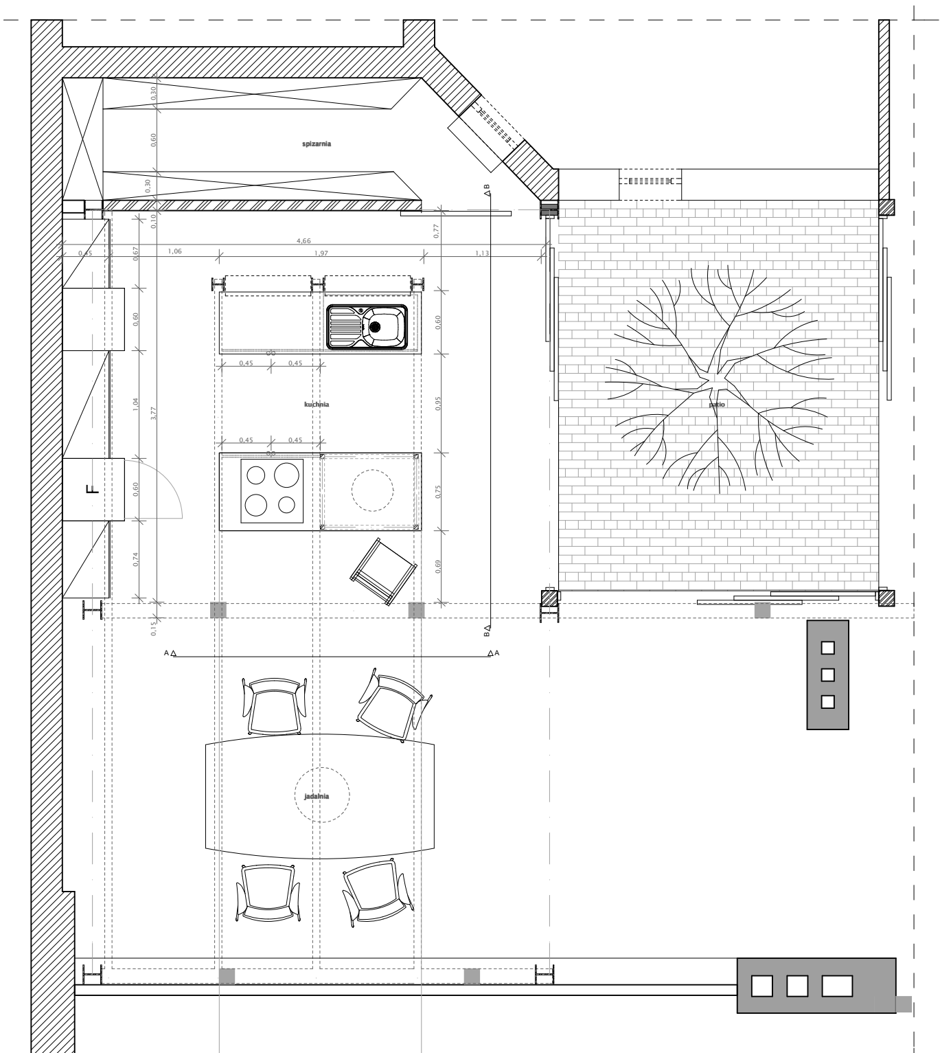
RZUT 1:50
