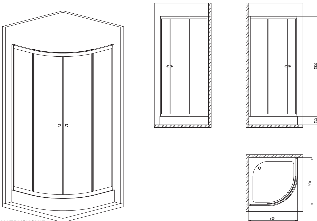
KABINY NATRYSKOWE Kabiny i brodziki Kabina Alfa KOD: KTA 051K
