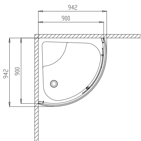
Wersja lewa - drzwi otwarte
